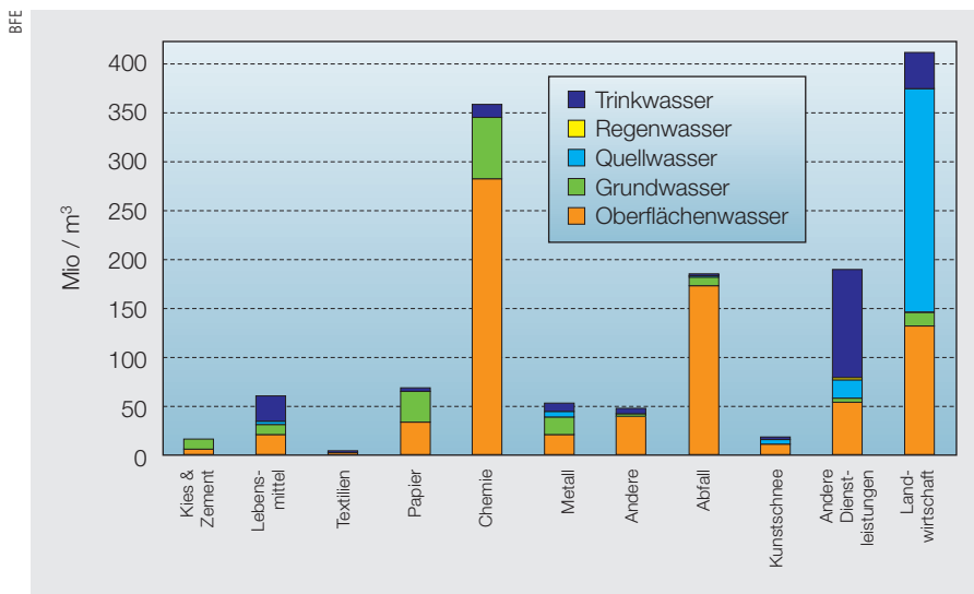
Grafik zum Wasserverbrauch verschiedener Branchen: Eine ökonomische Studie im Auftrag des BFE hat die Chemie-, Metall-, Papier- und Nahrungsmittelindustrie als potenzielle Standorte für thermomagnetische Generatoren identifiziert.
